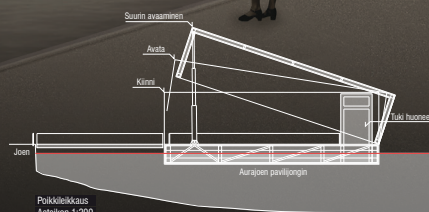
Poikkileikkaus Asteikon 1:200
