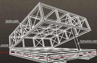
Rakenteellinen kaavio
