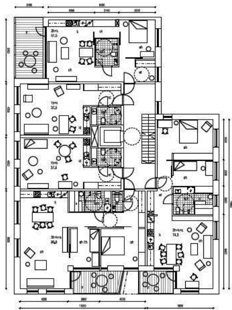
TYYPILLISET HUONEISTOPOHJAT 1/100
