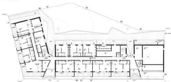
1. KERROS 1:200
