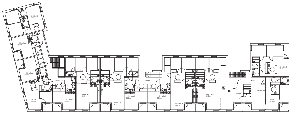
POHJAPIIRROS 1/200 5. KERROS (4.KRS SAMANLAINEN ILMAN SAUNAOSTAOT)
