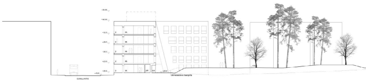
LEIKKAUS A-A 1/200
