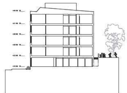
LEIKKAUS B-B 1:200
